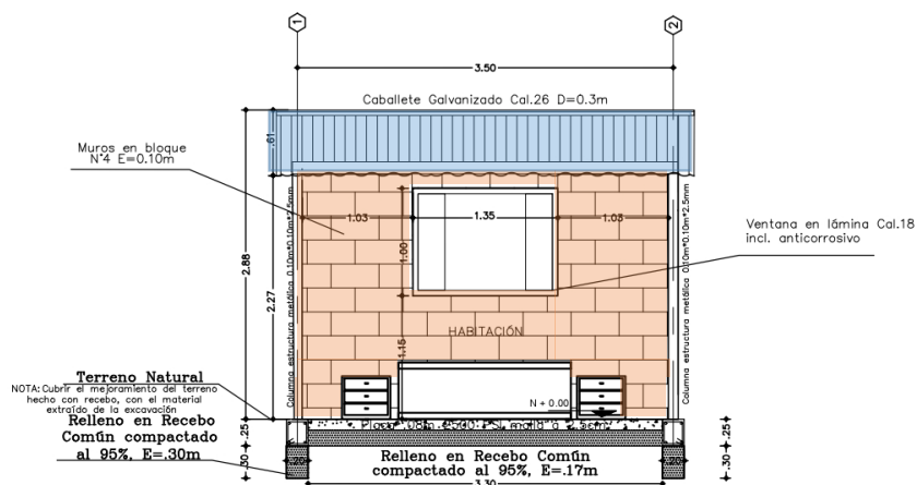
Vista fachada
