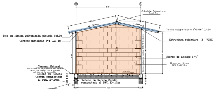
Vista fachada
