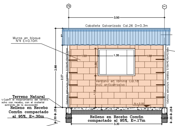
Vista fachada
